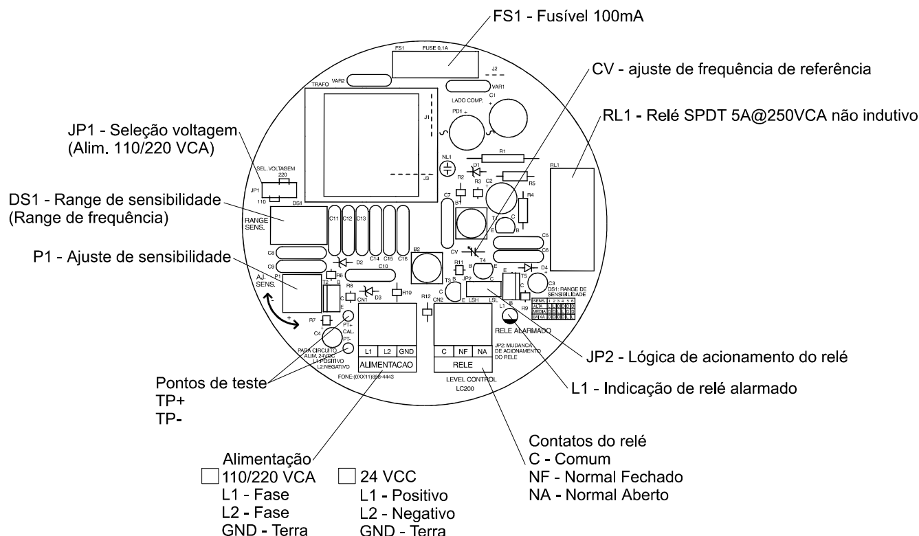
Figura 11 – Placa de circuito eletrônico.
